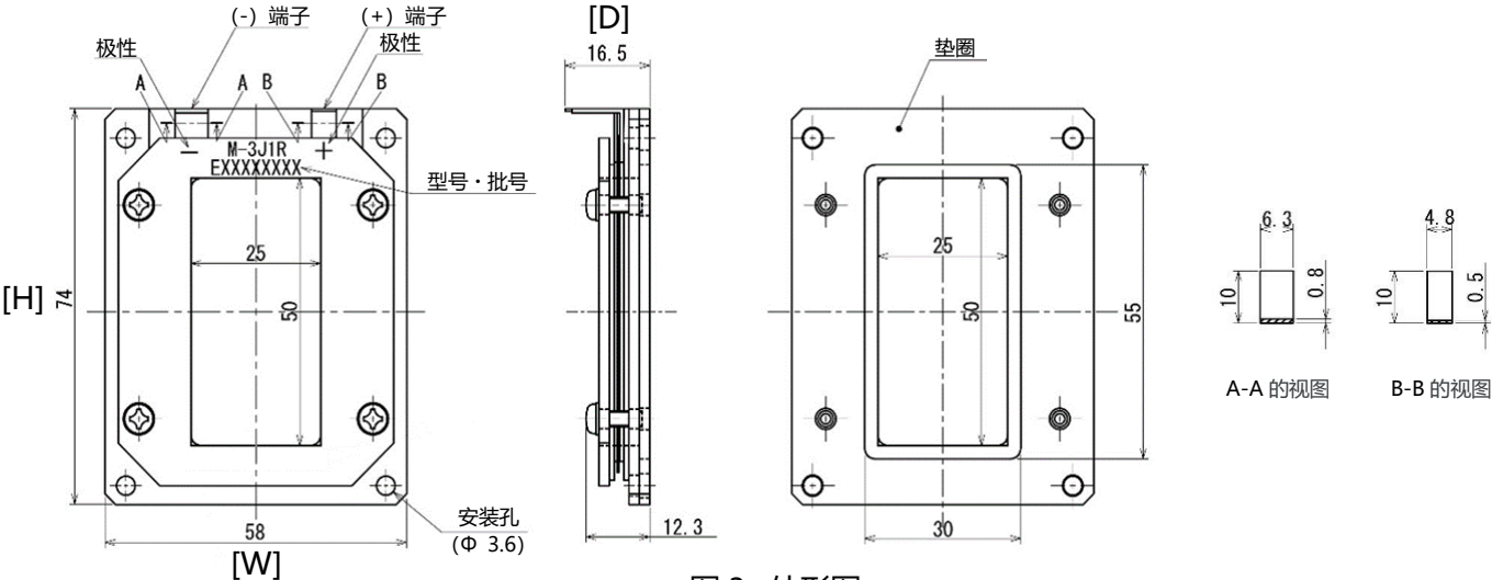
图 3. 外形图
