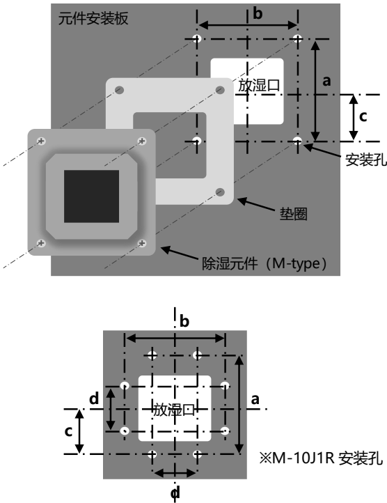
图 2. 安装示意图
